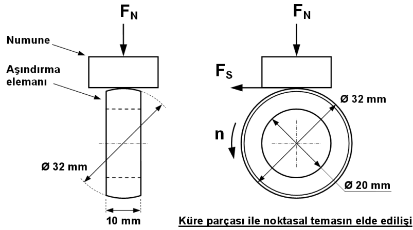
Şekil 4. Deneyde kullanılan pin-on-ring sistemi için temas geometrisi ve kuvvetler ( F_N normal kuvvet, F_S sürtünme kuvveti, n devir sayısı).
