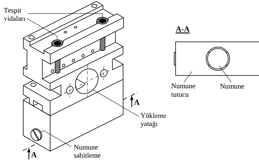
Şekil 6. Deneyde kullanılan numune tutucu.
