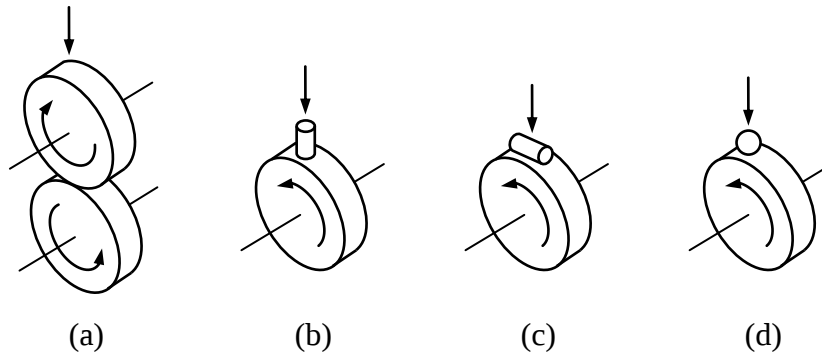
Şekil 3. TE 53SLIM çok-amaçlı sürtünme ve aşınma test cihazı ile uygulanabilen temas geometrileri: a) Ring-on-ring, b) Pin-on-ring, c) Block-on-ring, d) Ball-on-ring
