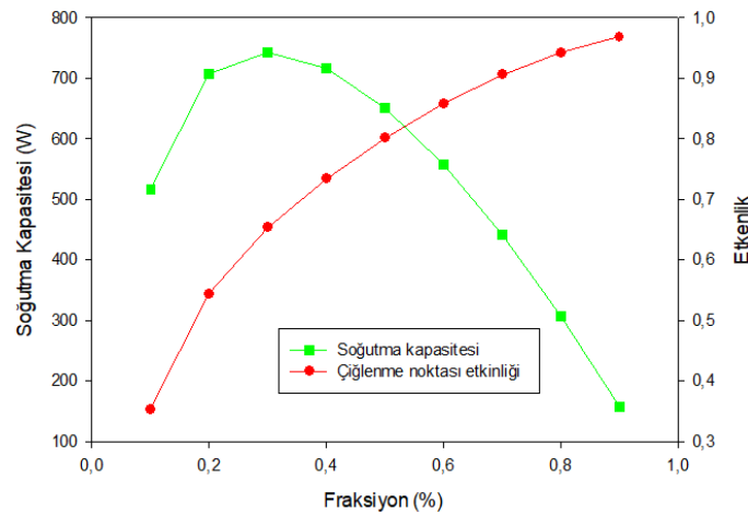
Şekil 11. Çalışma-giriş hava oranına ait soğutma kapasitesi ve etkinlik değerleri
