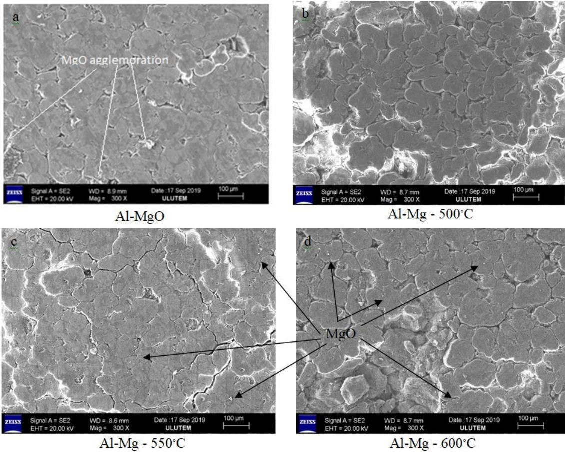
Şekil 2. Al-MgO kompozitinin 5 saat süreyle değişik sıcaklıklardaki sinterleme sonucu SEM yapıları a) Al-MgO, b) Al-MgO - 500°C, c) Al-MgO - 550°C, d) Al-MgO - 600°C
