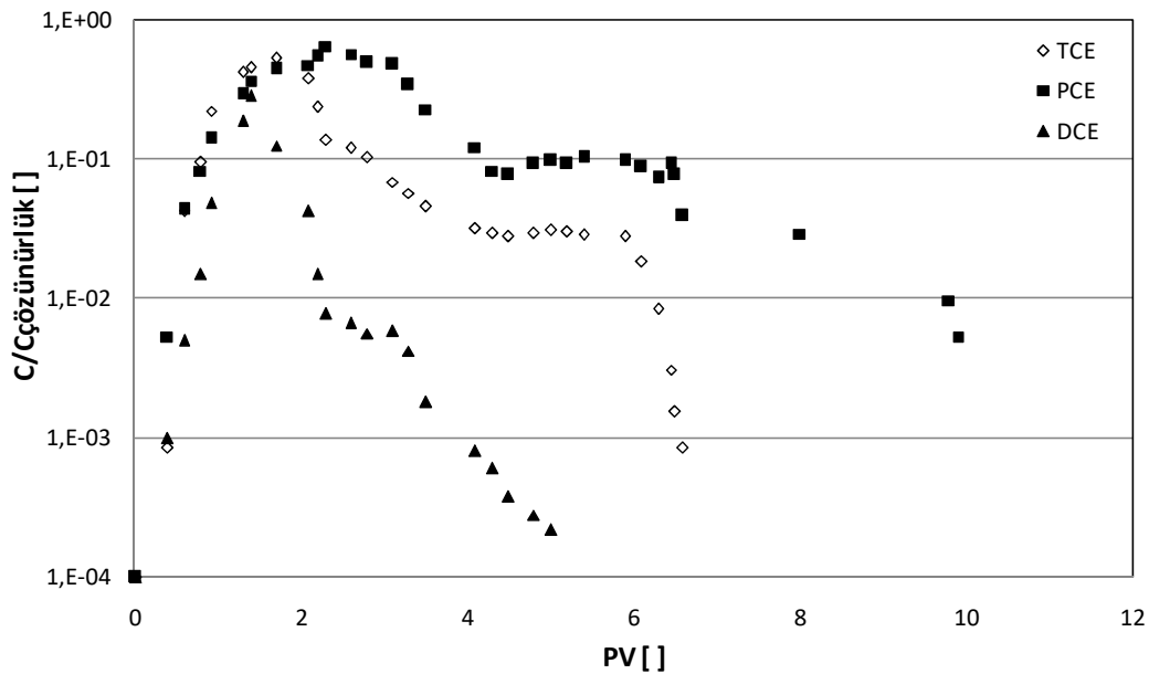
Şekil 5. Yüzey aktif maddeli (SDS) yıkama ile TCE, PCE ve DCE'nin zamana bağlı değişimi.
