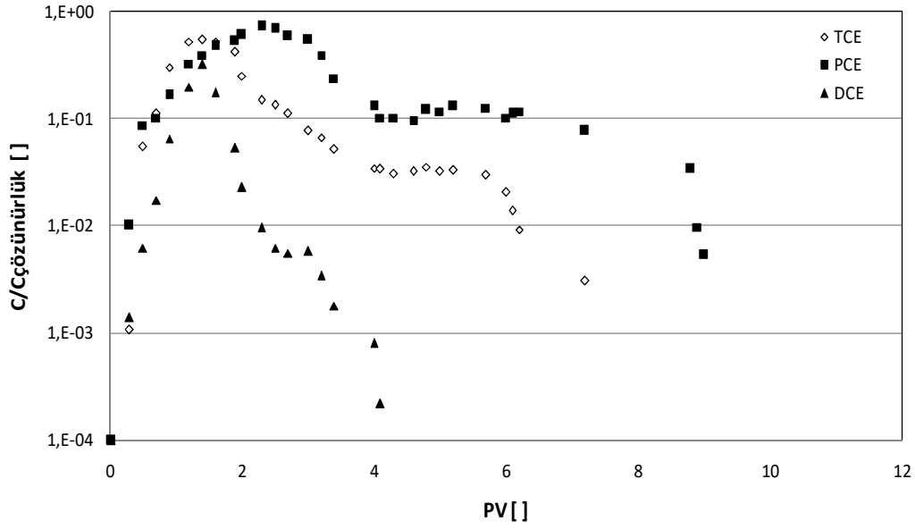
Şekil 4. Yüzey aktif maddeli (Tween80) yıkama ile TCE, PCE ve DCE'nin zamana bağlı değişimi (1PV=2,38saat)
