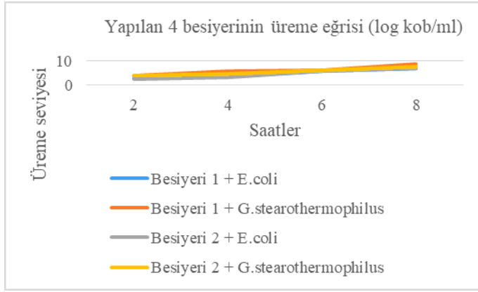
Şekil 3. Üreme eğrisi.
