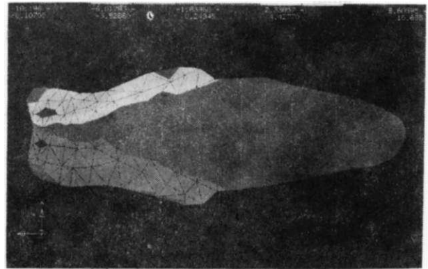
Grafik 1. 0° Tüberküllu modelde 10 kg.lık yükleme sonucu ortaya çıkan gerilim bölgeleri.
