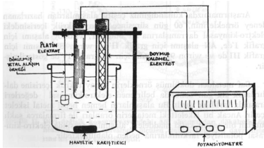
Resim 1. Araştırmamızda kullandığımız düzenek şematik olarak gösterilmiştir.
