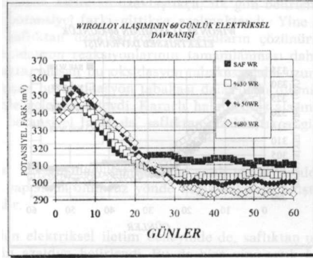
Grafik I. Dört değişik konsantrasyondaki wirolloy alaşımından dökülmüş örneklerin gözlem süresince ölçülen elektro-kimyasal davranışlarına ait veriler gösterilmiştir.
