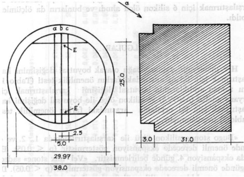
Şekil 1 : Boyutsal değişikliği ölçmede kullanılan paslanmaz çelik model.
