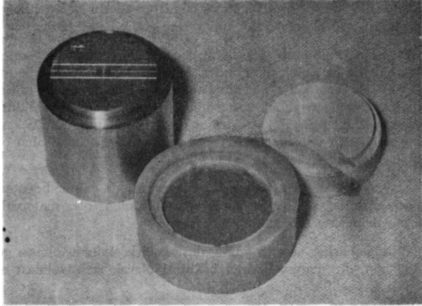
Resim 1 : Boyutsal değışikliğı ölçmede kullanılan paslanmaz çelik model, silikon ölçü ve alçı örnek.
