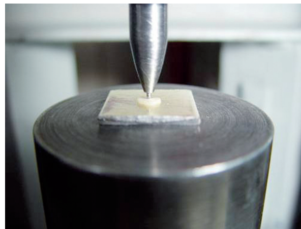
Resim 1. Universal test cihazında push-out testi uygulanması
