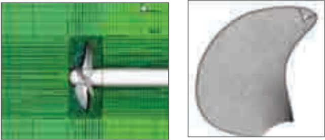
Şekil 4. Pervane üzerindeki sayısal ağ görünümü
