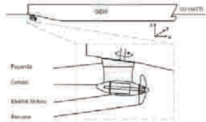
Şekil 1. Podlu pervane sistemi görünümü [7]
