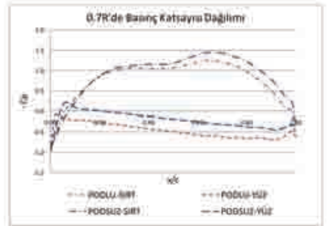
Şekil 22. 0.7 \times R pervane kesitinde podlu ve podsuz durumlar için basınç dağılımı ( C_p )
