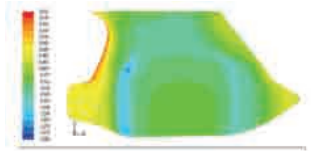
Şekil 16. Pervaneli durumda pod üzerindeki basınç dağılımı ( C_p )
