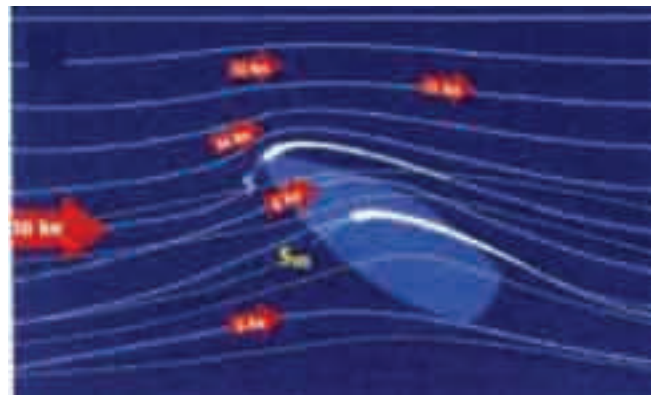
Şekil 14. İki adet yelken kullanımı gemiye tek yelkene göre daha büyük bir hız kazandırır. Mavi hatlar iki yelkene ait akım hatlarını sarı çizgiler tek yelken için akım hatlarını gösterir. [1]
