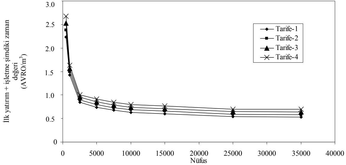
Şekil 4. Akdeniz suyu membran teknolojisi sistemlerinin farklı elektrik tarifelerine göre 1 m 3 üretilen su için toplam yatırım maliyetleri (Tarife-1 : 0.0967 €/kW (geçerli tarife); Tarife-2 : 0.1160 €/kW (% 20 artış), Tarife-3: 0.1354 €/kW (% 40 artış); Tarife : 0.1547 €/kW (% 60 artış))
