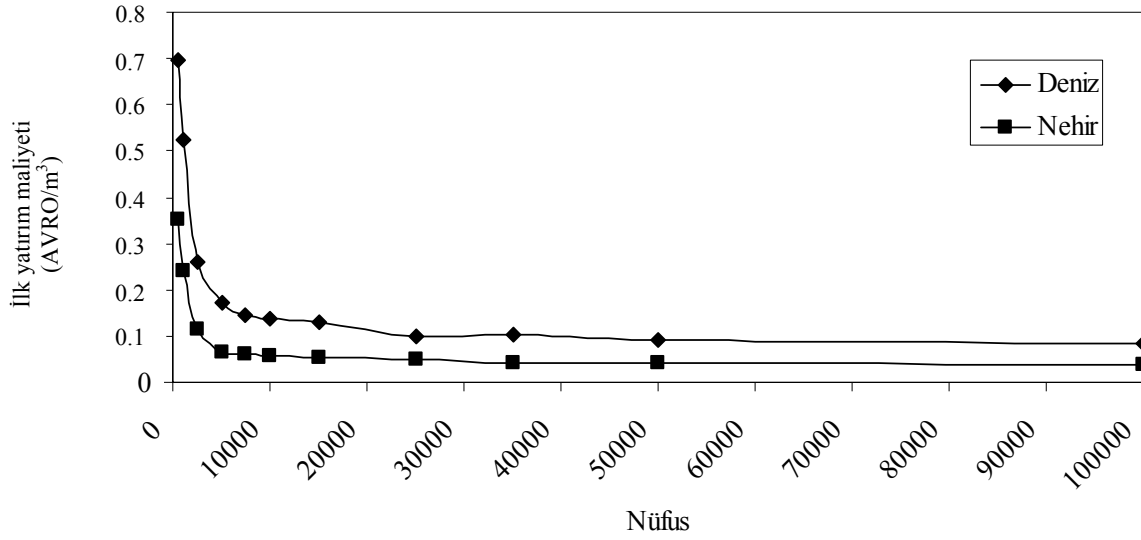
Şekil 7. Kızılırmak suyu ve Akdeniz suyu membran teknolojisi sistemlerinin bir (1) m³ üretilen su için ilk yatırım maliyetleri
