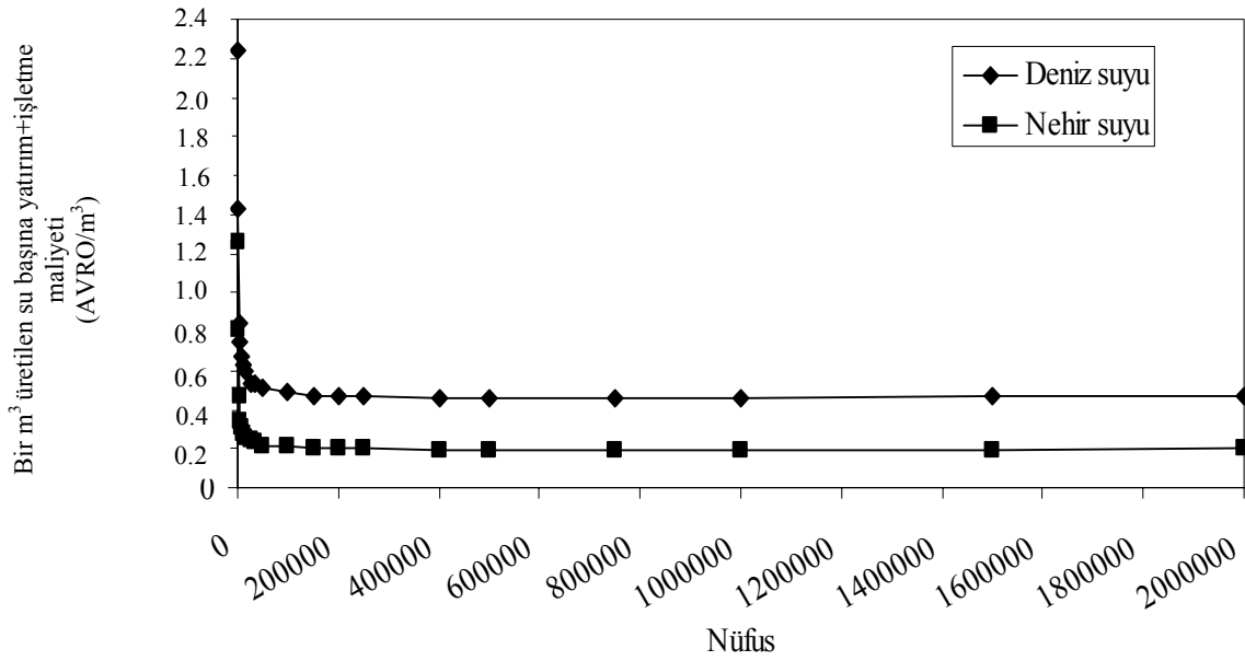
Şekil 8. Nüfusu 500-35000 arasında değişen yerlere hizmet eden nehir suyu ve Akdeniz suyu membran teknolojisi sistemlerinin 1 m³ üretilen su için toplam yatırım maliyetleri
