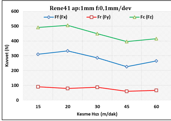
Şekil 2. Kesme hızı-Kesme kuvvetleri grafiği (Graphic of cutting speed-Cutting force)
