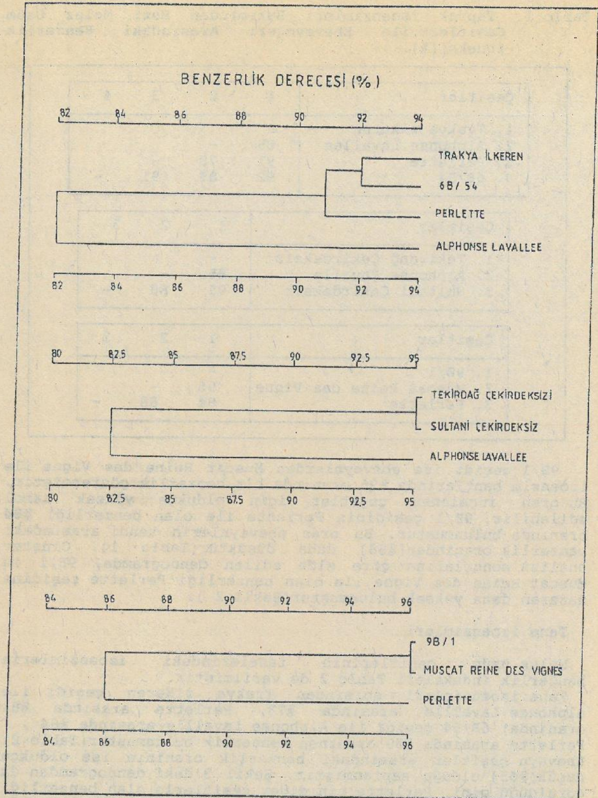
Şekil 2. Yaprak izoenzimleri açısından melezler ve ebeveynleri arasındaki farkları gösteren ve cluster analizi sonucunda elde edilen dendogram.
