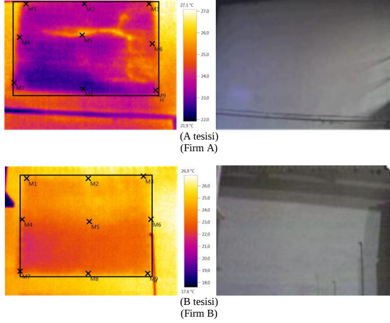
Şekil 5. Kurutma odası duvarının termal ve gerçek görüntüsü
