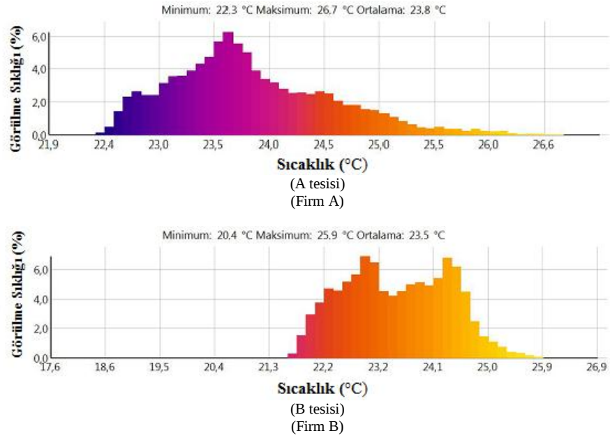
Şekil 6. Kurutma odası duvarının sıcaklık histogram grafiği
