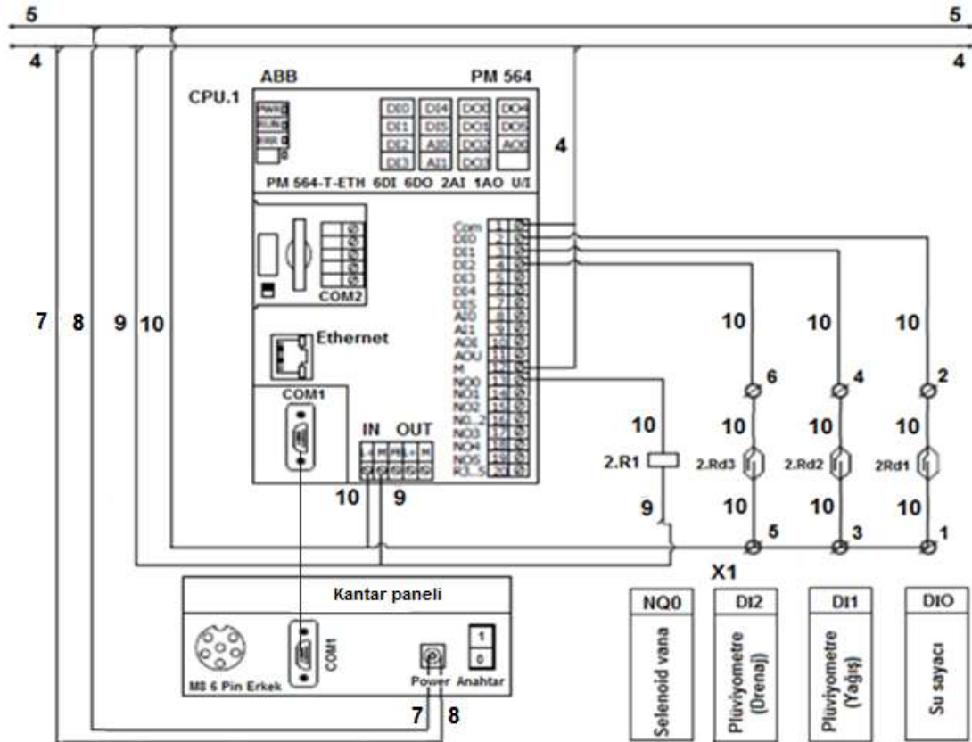
Şekil 3. Kantar, plüviyometreler, selenoid vana ve dijital su sayacı kontrol projesi.
