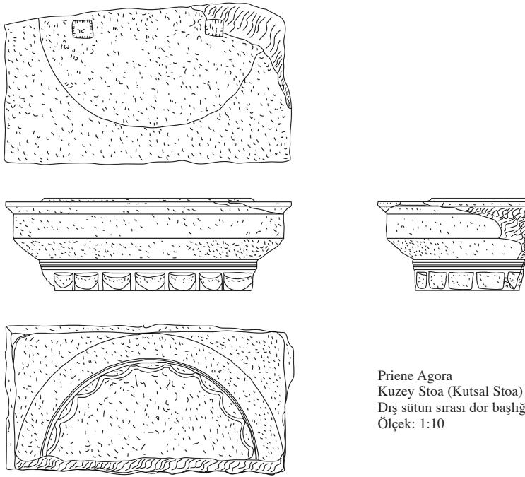
Fig. 24 Kutsal Stoa Dış Cephe Dor Başlığı Çizimi (Kienlin 2004a, Taf. 135'e göre).
