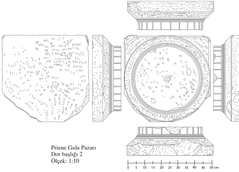
Fig. 23 Gıda Pazarı Kuzey Stoa dor başlığının çizimi (Çizim: K. Piechaczek'in çizimine göre).
