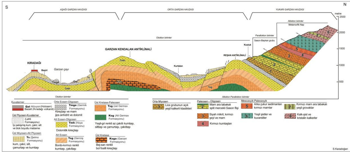
Şekil 4. Garzan Havzası'nın kuzeyi ve güneyi arasında geçirilmiş jeolojik-jeomorfolojik – tektonik kesit.
