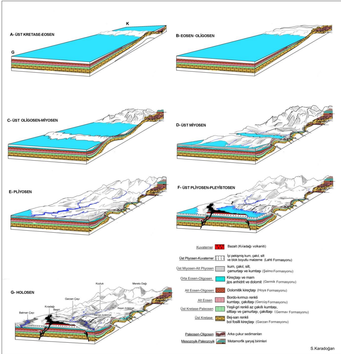
Şekil 8. Üst Kretase'den günümüze Garzan Havzası'nın jeomorfolojik evrimi.
