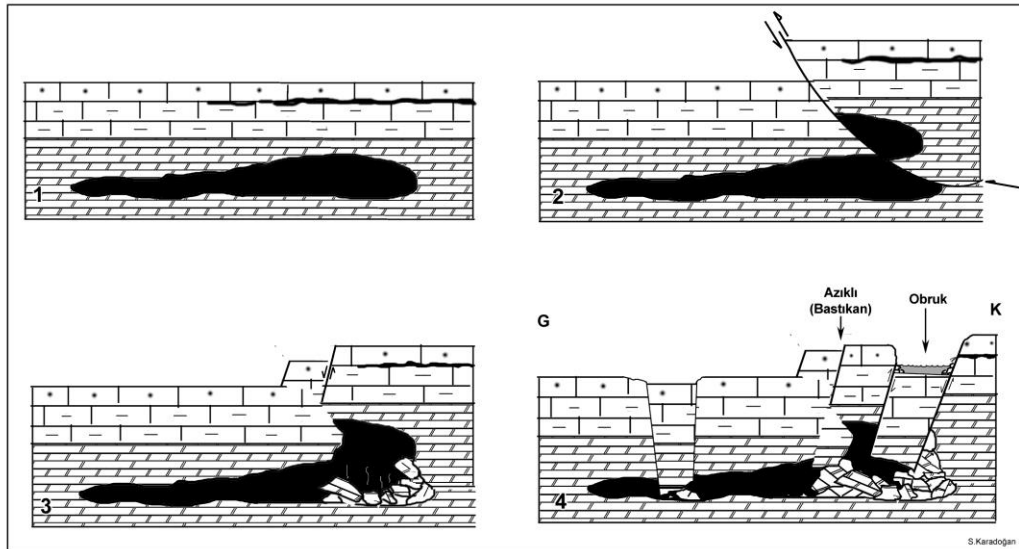
Şekil 11. Azıklı (Bastıkan) obruğunun oluşum aşamaları.
