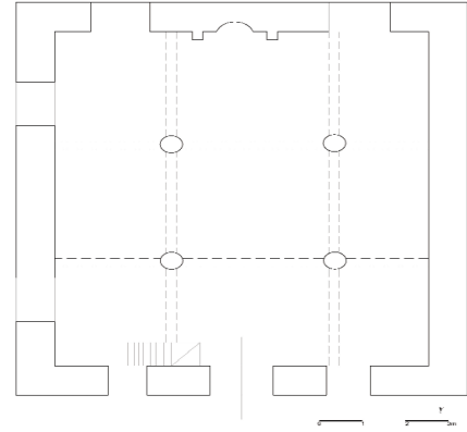
Çizim 8: Araköy Camii
