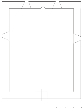
Çizim 11: Kale Köyü Camii
