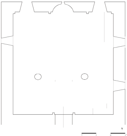
Çizim 5: Örenşar Camii
