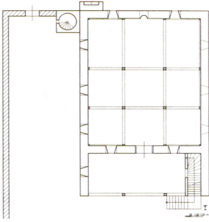
Çizim 1: Süleymaniye Mahallesi Camii
