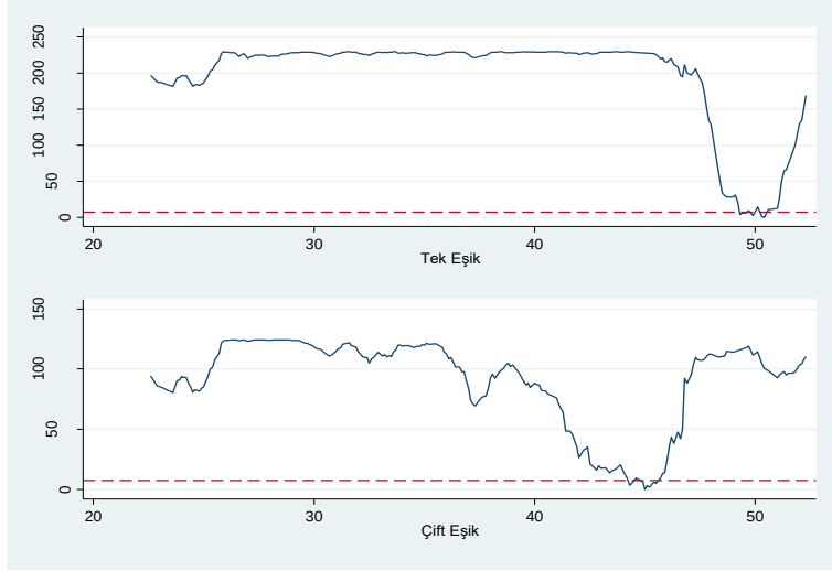
Şekil: 1 Tek ve Çift Eşik için LR En Çok Olabilirlik İstatistikleri
