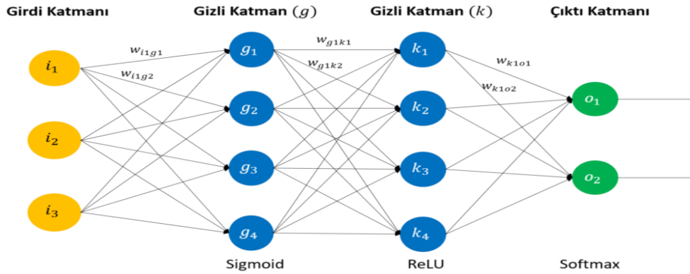
Şekil: 2 Geri Yayımlı Öğrenme Algoritması
