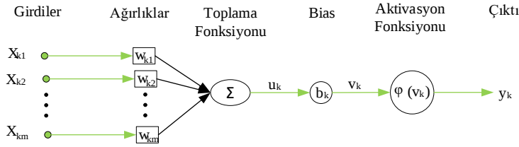
Şekil: 4 YSA'da Yer Alan Nöronların Genel Yapısı
