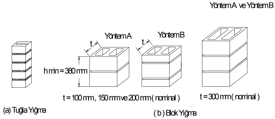
Şekil 2. Yığmanın eksenel basınç mukavemetini tayin etmek için kullanılan prizmalar [5].
