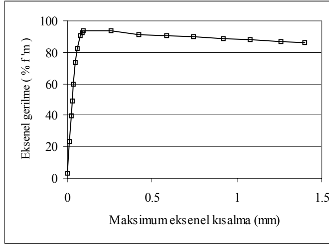
Şekil 13. Eksenel gerilme-maksimum eksenel kısalma eğrisi.
