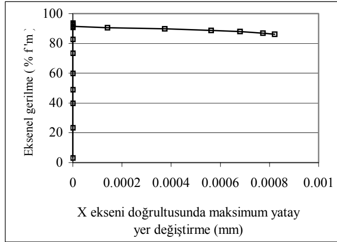
Şekil 14. X ekseninde maksimum yatay yer değiştirme ile eksenel gerilme eğrisi.
