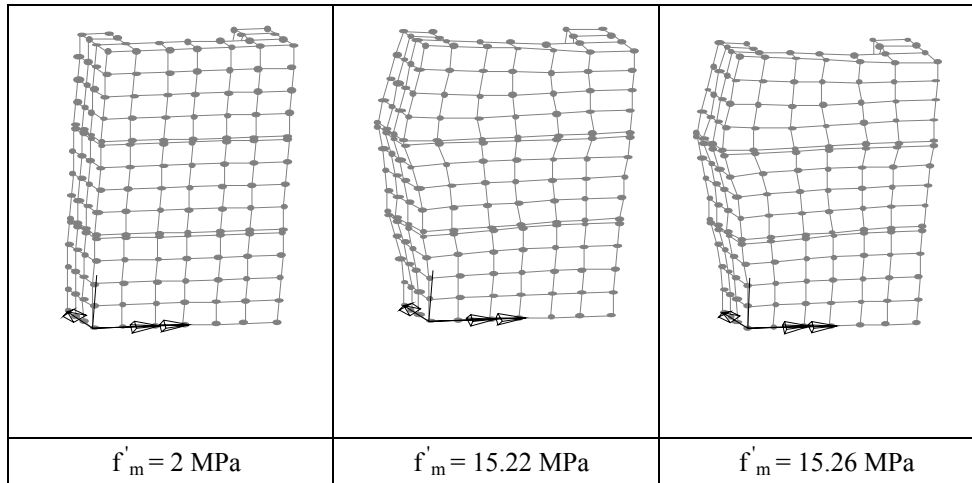
Şekil 8. Artan yük adımlarında prizmanın deforme şekilleri.
