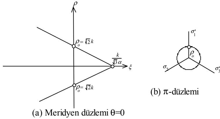
Şekil 5. Drucker-Prager kriteri [17].
