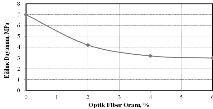
Şekil 7. Optik fiber içeriğine bağlı olarak eğilme dayanımının değişimi [9]
