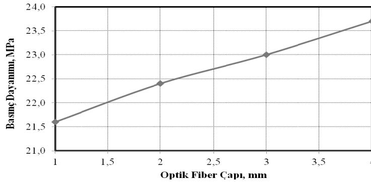
Şekil 5. Optik fiber çapına bağlı olarak basınç dayanımının değişimi [8]
