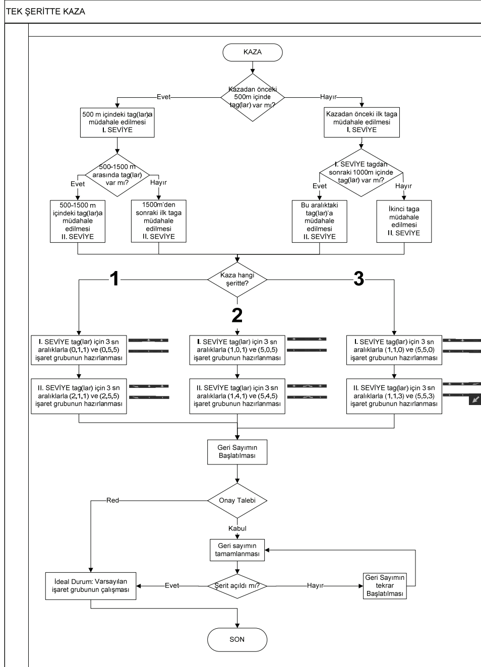
Şekil 5. Tek şeritte meydana gelen kazanın ŞKS akış şeması [11].
