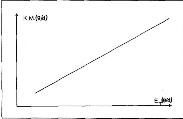
Şekil 6. Dört düz filament iplik örneği için young modülü kopma mukavemeti büyüklüklerinin değişimini gösteren lineer regresyon analizi grafiği
