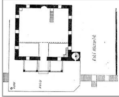
Şekil 4: Bozhane Köyü Camii'nin Planı
