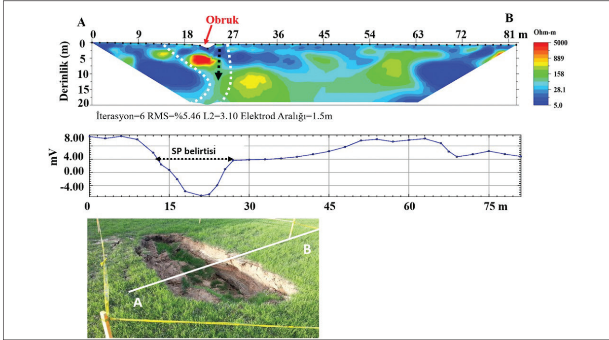
Şekil 14. Obruk üzerinde alınan öz direnç (a) ve SP (b) ölçümlerine ait kesitler. Obruğun lokasyonu öz direnç profili üzerinde verilmektedir. Yüksek ve düşük öz direnç anomalilerinin birleştiği alanda belirgin bir SP anomali gözlemlenmektedir. Öz direnç kesitinde verilen kesikli siyah ok, obruğun altındaki toprağın kayabileceği doğrultuyu ifade etmektedir. (c) de ise obruğun fotoğrafı ve ölçüm alınan AB profili gösterilmektedir.
