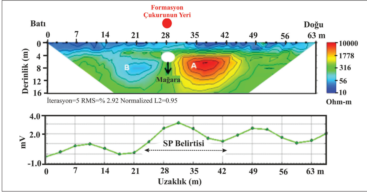
Şekil 16. (a) L1 profili boyunca alınan öz direnç ölçümlerinden elde edilen kesit. Formasyon Çukuru'nun lokasyonu kırmızı, mağaranın lokasyonu ise beyaz dolgu daire ile temsil edilmiştir. (b) L1 profili boyunca elde edilen SP değerleri. En yüksek SP potansiyel değerinin gözlemlendiği lokasyon ile mağaranın lokasyonu iyi bir korelasyon göstermektedir.
