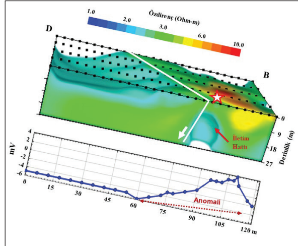
Şekil 9. (a) Üç boyutlu (3B) özdirenç yapma- kesiti ve (b) SP profili Zilker Park'ın güneyinde bir iletim hattı ve olası fay anomalisinin olduğunu göstermektedir. Kırmızı yıldız sembolü, havuzun güney kapı girişinin yaklaşık olarak konumunu göstermektedir. Şekillerin yönü, anomalilerle uyumlu olması adına batı-doğu'dan ve doğu-batı'ya çevrilmiştir.
