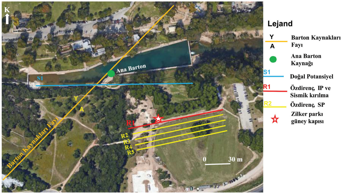
Şekil 6. Barton Yüzme havuzunun güneyindeki özdirenç, SP, IP ve sismik kırılma çalışmalarının lokasyonlarını gösteren havadan bir harita. Bu çalışmada sadece özdirenç profili R1” tartışılmıştır. R2 ile R5 arasındaki özdirenç profillerine ait sonuçlar Saribudak vd., 2013 ve Saribudak ve Hauwert, 2017’de yer almaktadır.
