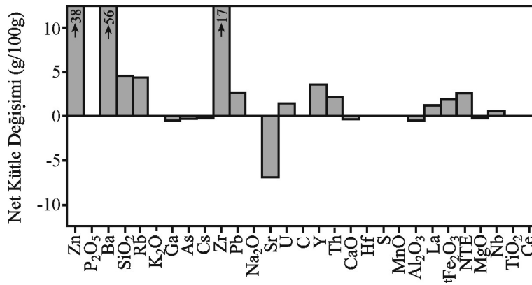
Şekil 13. Dasit-II'den alınan örneğin (Cm) az alterasyona uğramış kayaca göre net kütle değişimi.
