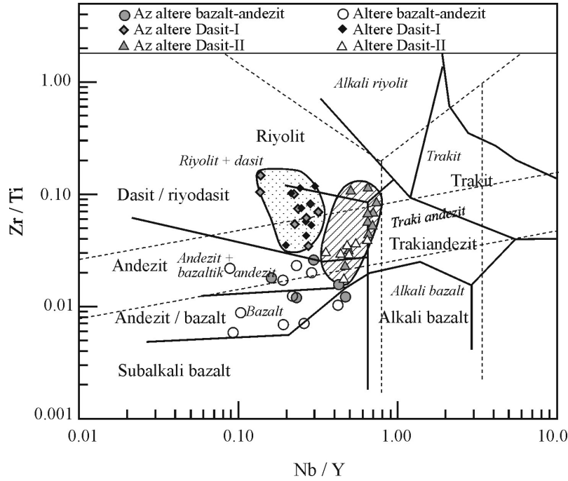
Şekil 4. Zigana Volkanitleri'nin Nb/Y'a karşı Zr/TiO 2 x0.0001 (Winchester ve Floyd, 1977'den değiştirilerek Pearce, 1996) diyagramında sınıflandırılması. Veriler Sipahi (2005)'den alınmıştır.
