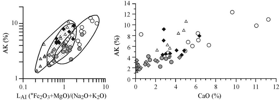
Şekil 5. Zigana Volkanitleri'nin AK'ya karşı alterasyon indeksi ( L_{AI} = \text{Fe}_2\text{O}_{3\text{toplam}} + \text{MgO} / (\text{Na}_2\text{O} + \text{K}_2\text{O}) ) ve CaO diyagramındaki dağılımları. Semboller Şekil 4 ile aynıdır.
