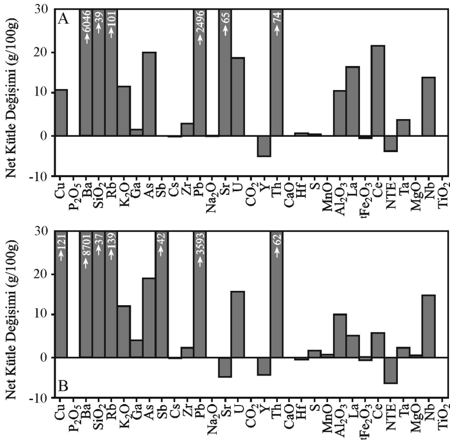
Şekil 12. Az altere Dasit-I'ten çok altere Dasit-I'e doğru alınan örneklerdeki net kütle değişimleri. A) Alterasyona uğramış kayaç (örnek D4+D6), B) Çok alterasyona uğramış kayaç (örnek D1).
