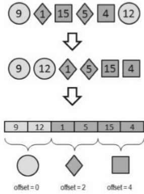
Şekil 12 – Geometri Örnekleme Aşamaları (Johansson M.,2013)
