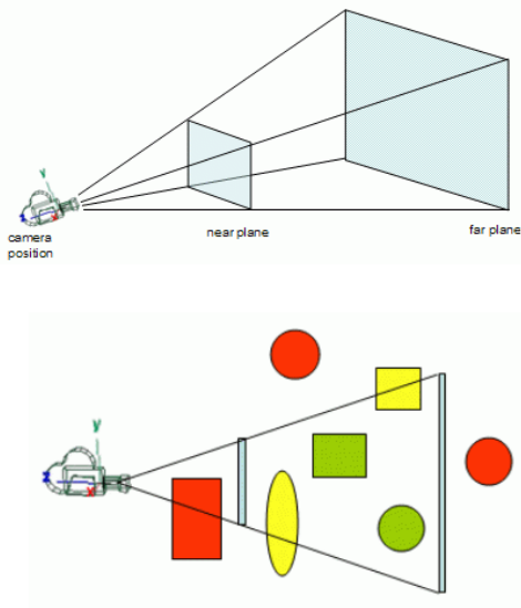
Şekil 7 – VFC (View Frustum Culling) Sistemi (URL-3)
