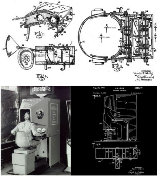
Şekil 1- Sensorama,1962 (URL-1)
