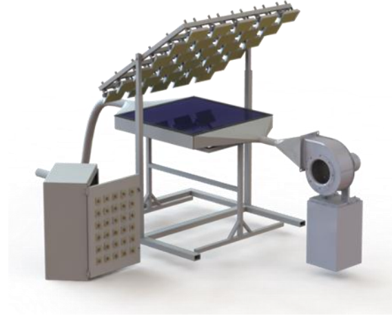
Şekil 1. Deney Düzeneği
