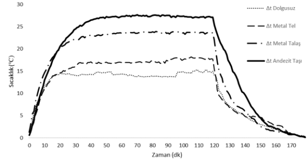
Şekil 9. 1,2 m/s hava hızındaki \Delta t değerlerinin grafiksel görünüşleri
