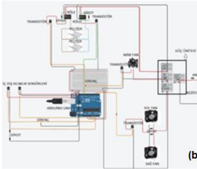
Şekil 3. Akıllı masa için elektronik devre tasarımı a) proteus simülasyon b) devre şeması
