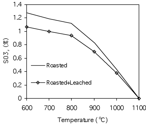
Figure 8: Effects of roasting and leaching after roasting on reduction of sulphur content Şekil 8: Kavurma ve kavurma sonrasında liç işlemlerinin kükürt içeriğindeki azalmaya etkileri
