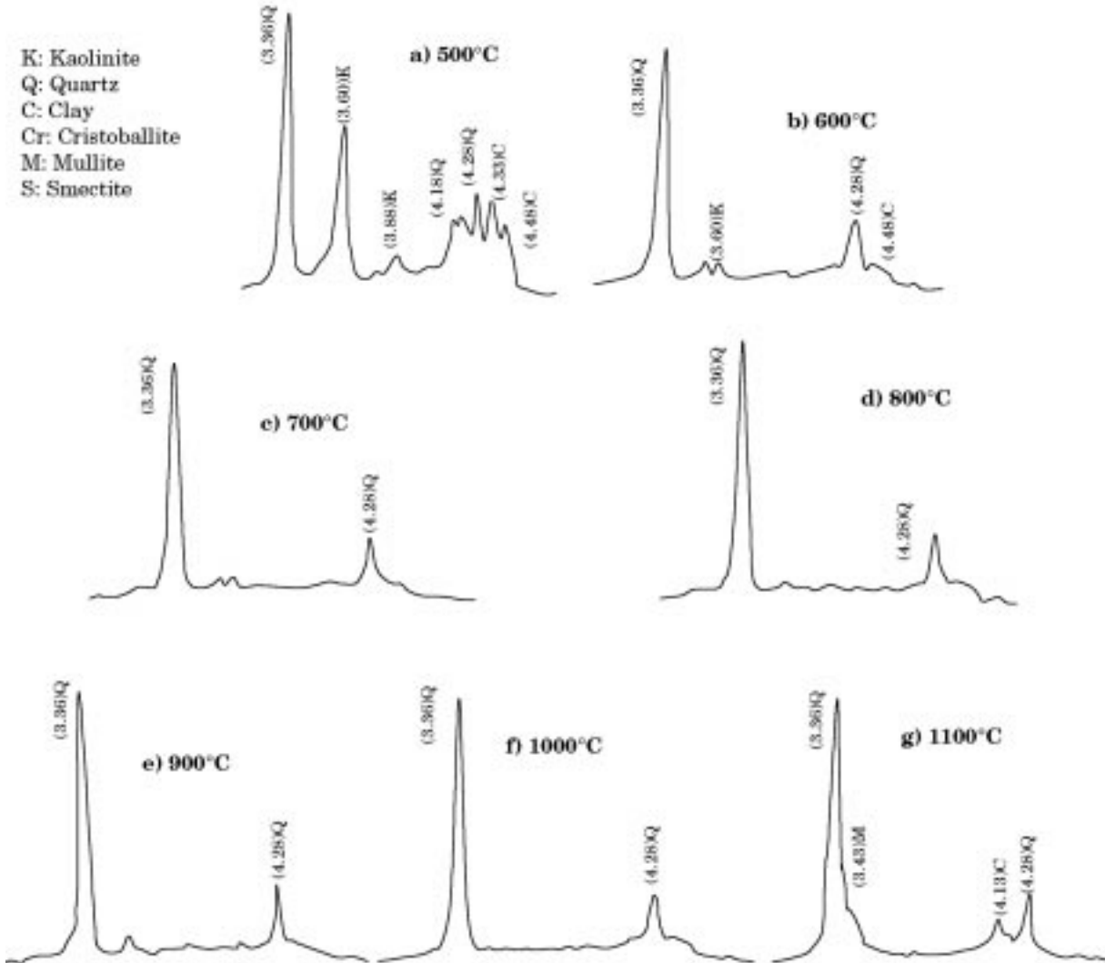
Figure 9: XRD patterns of roasted samples at different temperatures Şekil 9 : Farklı sıcaklıklarda kavurulmuş numunelerin X-ışını kırınimleri
