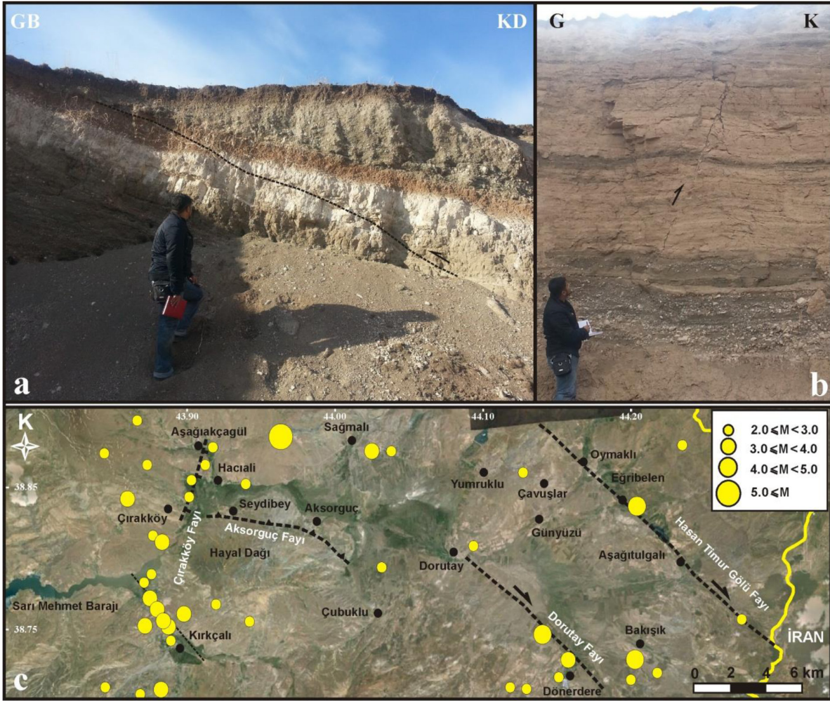
Şekil 3. Dorutay Havzası gölsel çökellerinde belirlenen; bindirme fayı (a) ve ters fay (b). Dorutay Havzası ve yakın çevresinde aletsel dönemde meydana gelmiş olan M=2 ve üzeri büyüklüklerdeki depremlerin (KOERI, 2014) dış merkezlerini gösteren Google Earth uydu görüntüsü (c).
