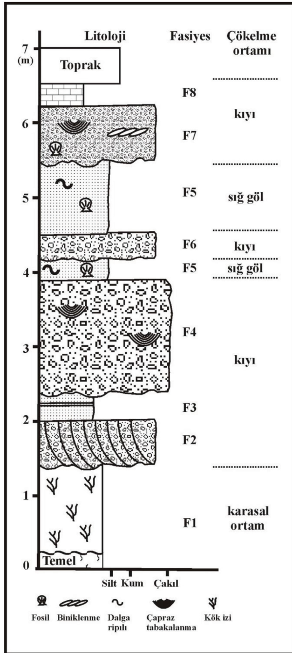
Şekil 5. Sedimanter fasiyeslerin dizilimlerini ve çökelme alt ortamlarını gösteren ölçülü stratigrafik istif.
