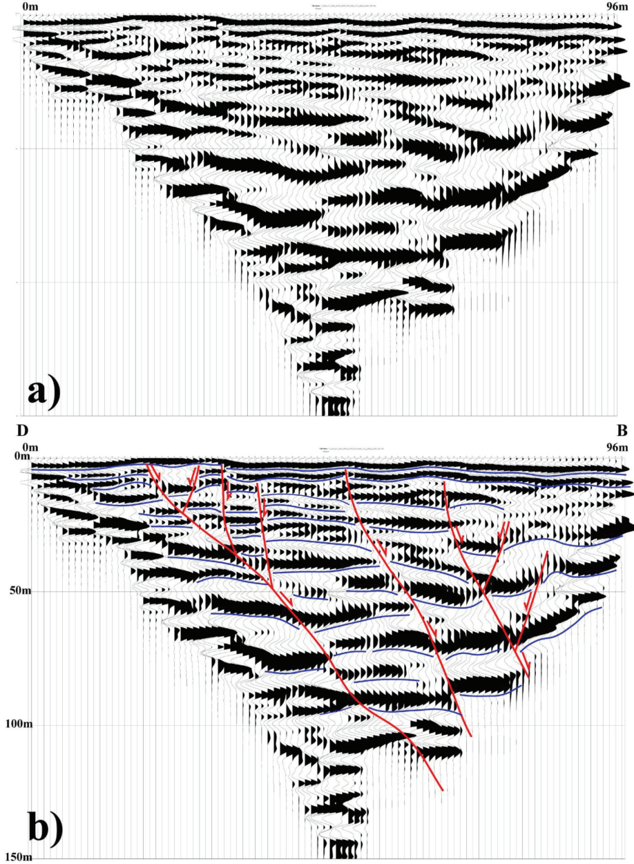
Şekil 12. Başayaş sismik yansıma kesiti (B1 hattı): a) yorumlansuz, b) yorumlanmış. Konum için Şekil 3'e bakınız. Figure 12. Başayaş seismic reflection section (B1 line): a) uninterpreted, b) interpreted. See Figure 3 for location.
