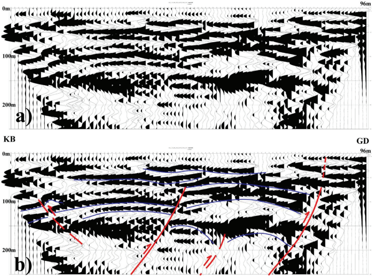
Şekil 11. Mülk-ek ova sismik yansıma kesiti (M3 hattı): a) yorumluz, b) yorumlanmış. Konum için Şekil 3'e bakınız. Figure 11. Mülk-addition (plain) seismic reflection section (M3 line): a) uninterpreted, b) interpreted. See Figure 3 for location.
