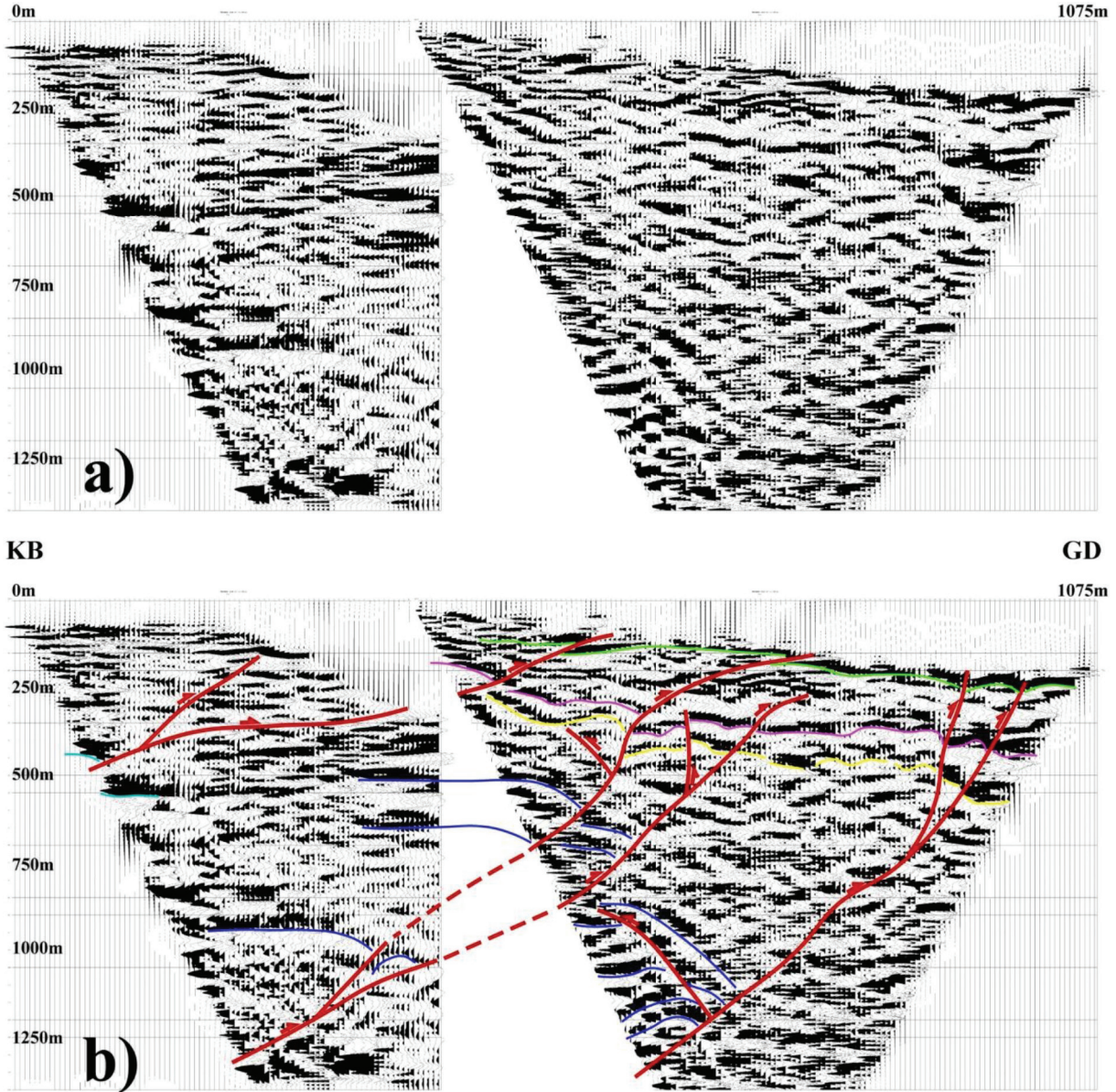
Şekil 9. Mülk sismik yansıma kesiti (M1 hattı): a) yorumluz, b) yorumlanmış. Konum için Şekil 3'e bakınız. Figure 9. Mülk seismic reflection section (M1 line): a) uninterpreted, b) interpreted. See Figure 3 for location.
