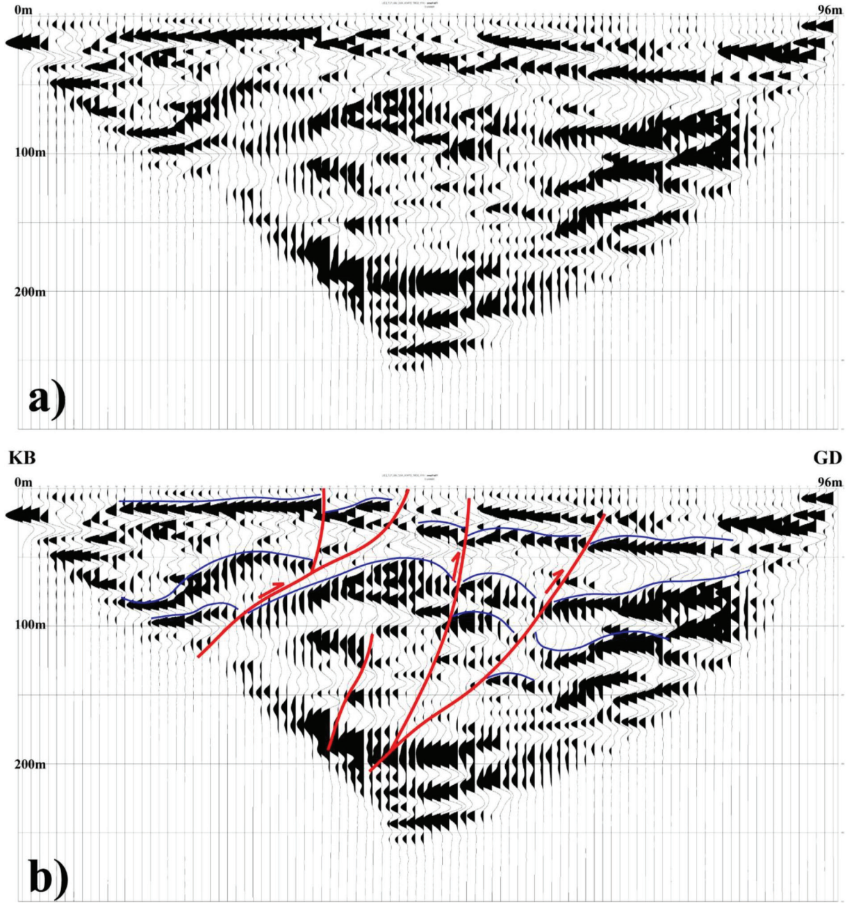
Şekil 10. Mülk-ek kenar sismik yansıma kesiti (M2 hattı): a) yorumlansız, b) yorumlanmış. Konum için Şekil 3'e bakınız.
