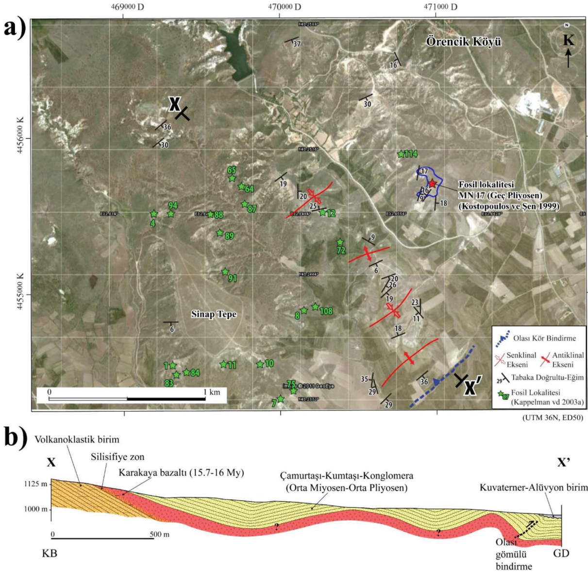
Şekil 15. a) Üzerinde yapısal unsurların gösterildiği, AKTK'nin kuzeydoğu devamındaki Sinap Tepe civarının Google Earth görüntüsü. Konum için Şekil 1a'ya bakınız. Yeşil yıldızlarla gösterilen fosil lokaliteleri 9.3 ile 10.9 My yaş aralığındadır (Kappelman vd., 2003a). b) Neojen birim tabakalarındaki olası kör bindirmeye ilişkili kıvrımlanmayı gösteren jeolojik enine kesit. Kesit hattının konumu için Şekil 15a'ya bakınız.
