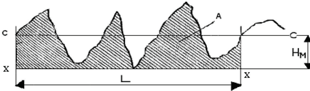
Şekil 2. Ölçüm yapılan yüzeyin profili Fig.2. Profile of measuring surface
