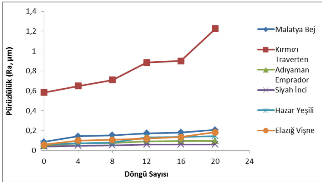
Şekil 4. Termal yaşlandırma deneylerinde döngü sayısına göre pürüzlülük değişimleri Figure 4. Roughness changes with respect to cycle number in the thermal ageing test
