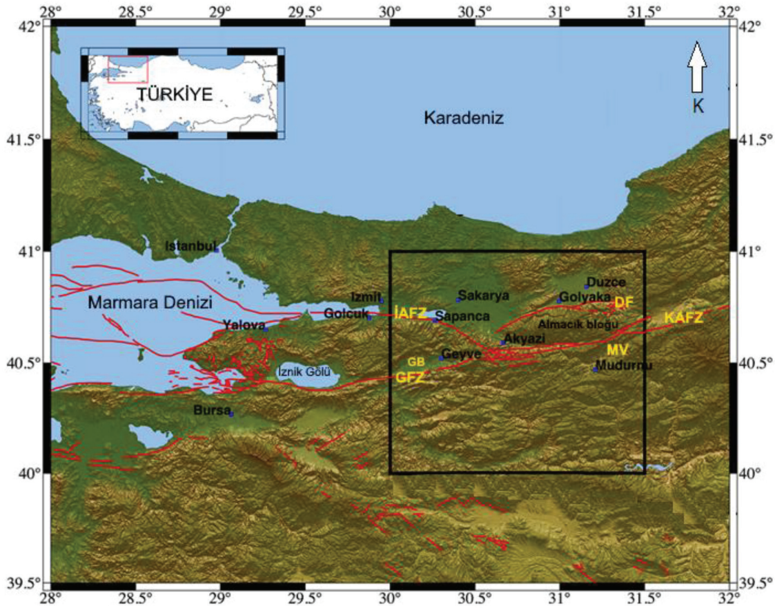
Şekil 1. Doğu Marmara bölgesinde yer alan çalışma alanı. KAFZ'nin kuzey ve güney kolları Maden Tetkik Arama (MTA) kurumu tarafından sunulan güncel fay haritasından (Saroglu vd., 1992) derlenmiştir. (İAFZ: İzmit-Adapazarı Fay Zonu, DF: Düzce Fayı, MV: Mudurnu Vadisi, KAFZ: Kuzey Anadolu Fay Zonu, GB: Geyve Baseni, GFZ: Geyve Fay Zonu)
