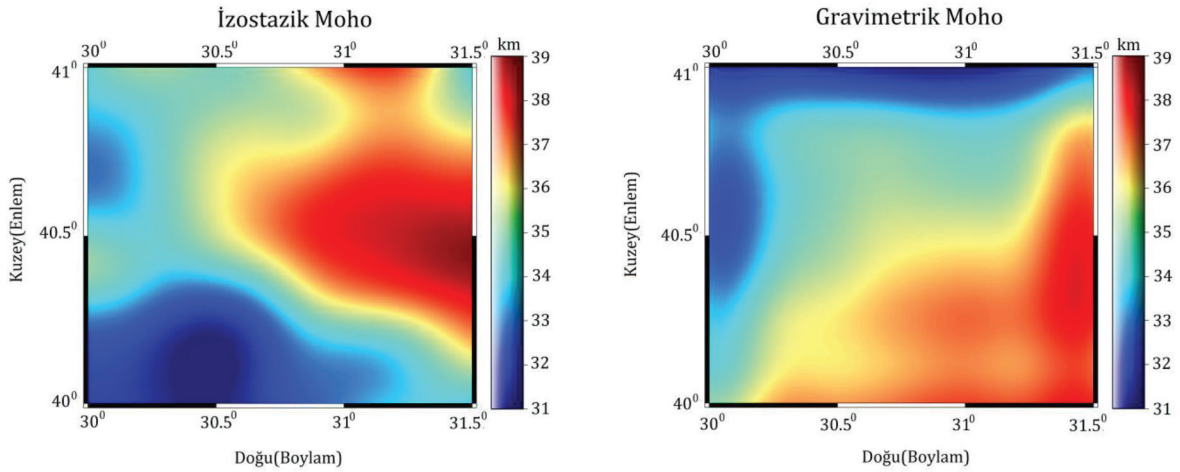
Şekil 6. Vening-Meinesz modeline göre kestirilen izostazik Moho haritası (solda) ve Parker-Oldenburg ters çözüm algoritmasıyla kestirilen gravimetrik Moho haritasının (sağda) karşılaştırılması (Sönmez, 2015).
