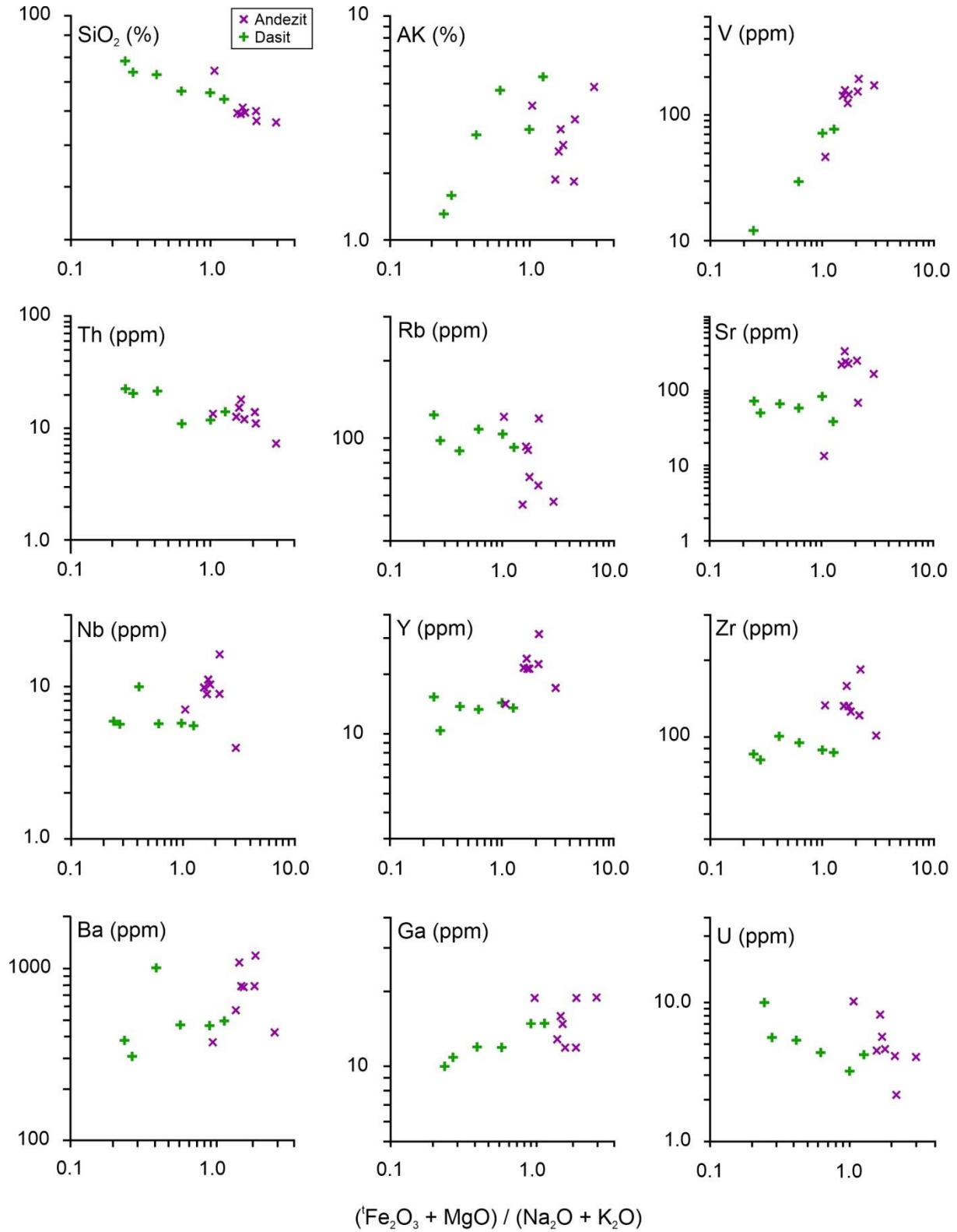
Şekil 10. Andezit ve porfirik dasit dayklarında bazı iz elementlerinin (ppm), L_{AI}(Fe_2O_3+MgO)/(Na_2O+K_2O) oranına karşı değişim diyagramları.
