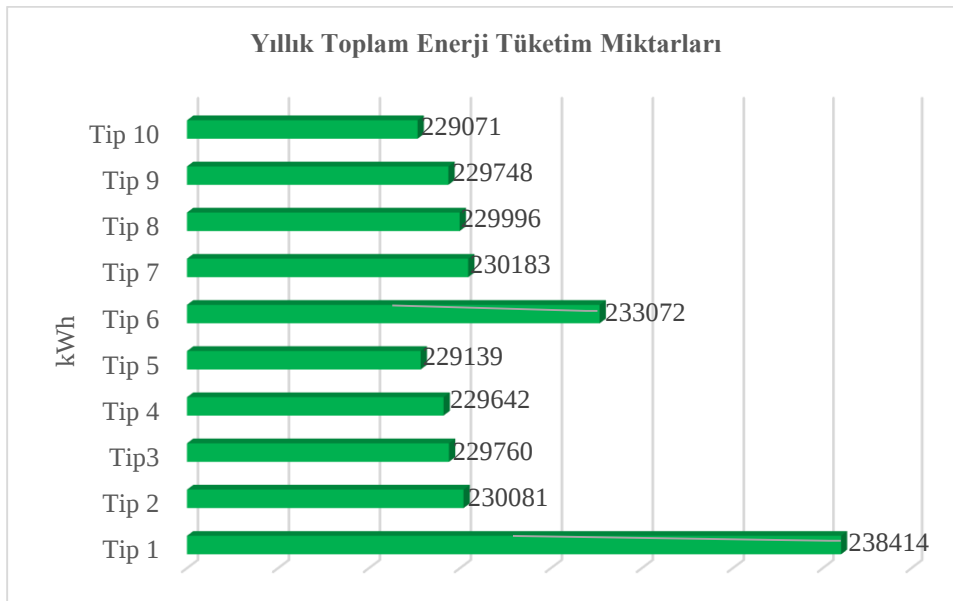
Şekil 12. Yıllık toplam enerji tüketim miktarları
