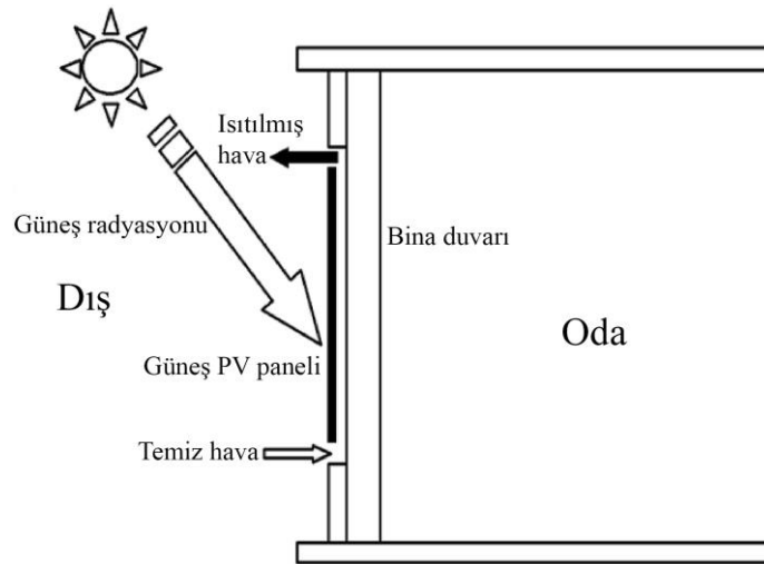
Şekil 4. Fotovoltaik trombe duvar
