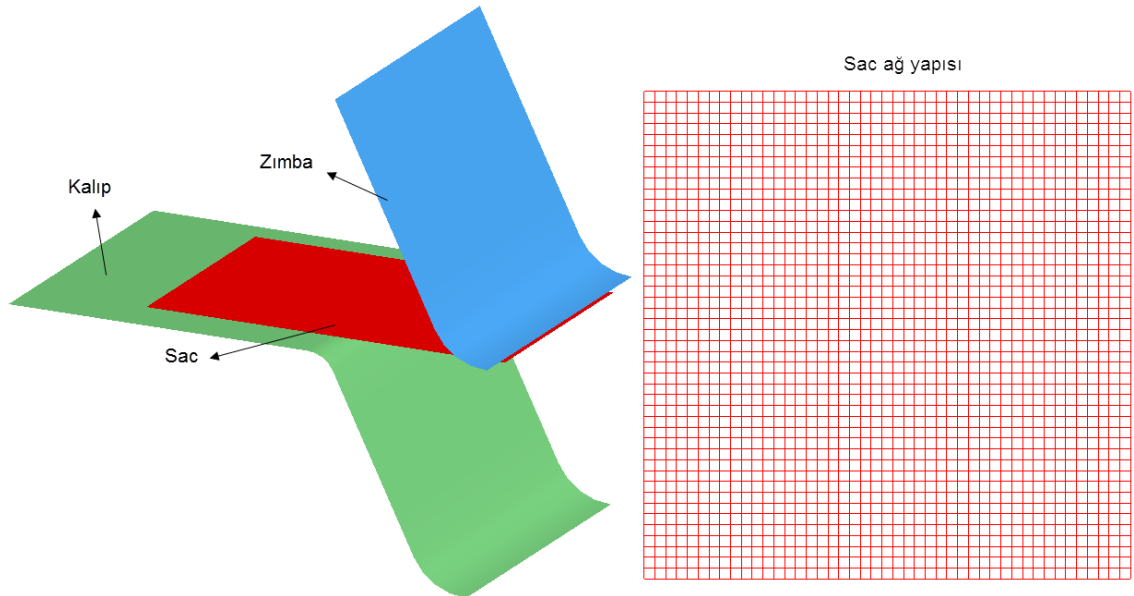
Şekil 6. V-kalıpta eğme sonlu elemanlar modeli ve sac açınım ağı yapısı
