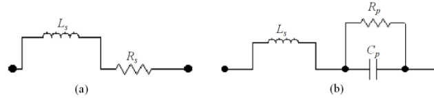
Şekil 2. HPND-4028 diyotunun eşdeğer devre modeli. (a) Pin diyot iletimde. (b) Pin diyot kesimde.
