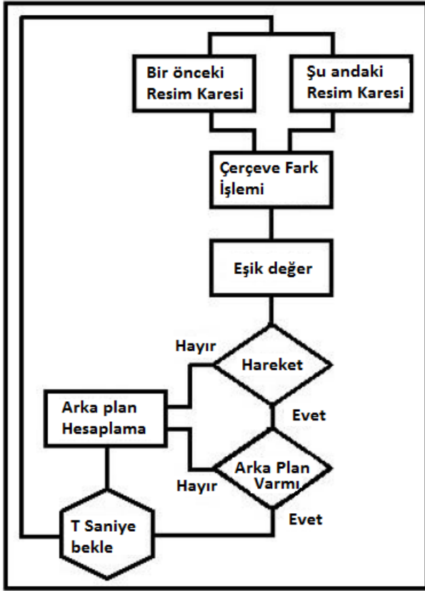
Şekil 4. Arka Plan Ayrımı için Çerçeve Fark Algoritması Akış Şeması.
