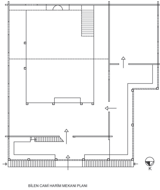
Çizim 2: Bilen Köyü Camii Harım Mekânı Planı
