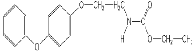
Şekil 1. Fenoksikarb: C_{17}H_{19}NO_4
