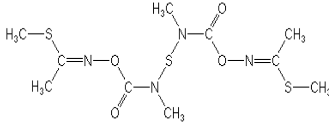
Şekil 2. Thiodicarb: C_{10}H_{18}N_4O_4S_3
