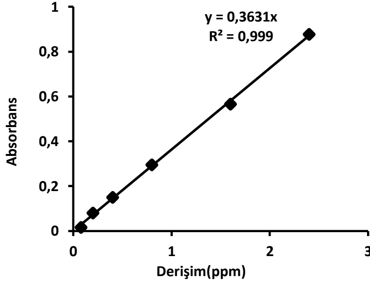
Şekil 7. 0,08-2,4 \mu\text{g mL}^{-1} arasında değişen Ponceau 4R derişimi, pH 6-9, 2,000 \text{ Na}_2\text{SO}_4 , %10 Brij 58, 70^\circ\text{C} ' de 10 dakika süreyle inkübasyon
