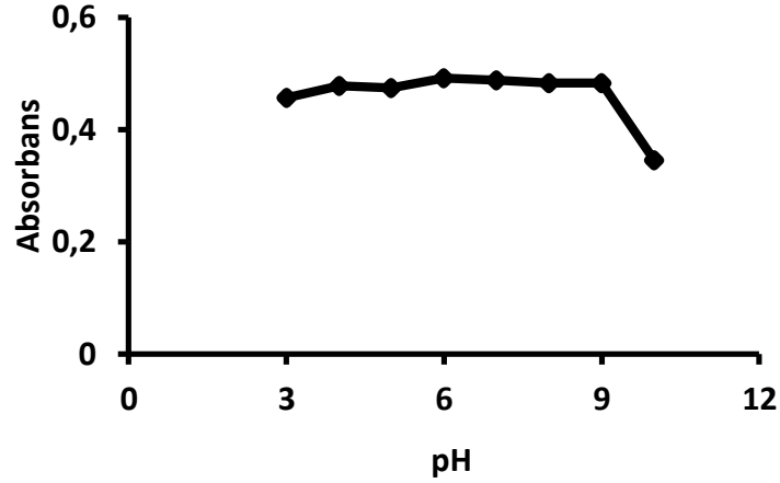
Şekil 3. pH'nın ekstraksiyon verimliliği üzerine etkisi. 2,4 \mu\text{g/mL} Ponceau 4R, %10 Brij 58, 2,000 g \text{Na}_2\text{SO}_4 , 70°C' de 10 dakika süreyle inkübasyon.
