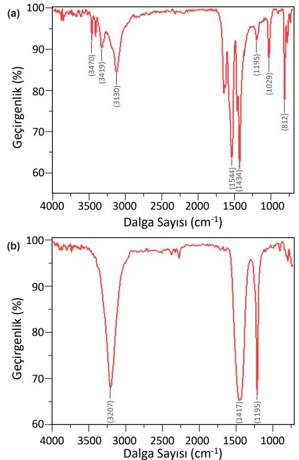
Şekil 1. a). Melamin FTIR grafiği, b). Borik asit FTIR grafiği (FTIR graph of a). FTIR graph of melamine, b). FTIR graph of boric acid).
