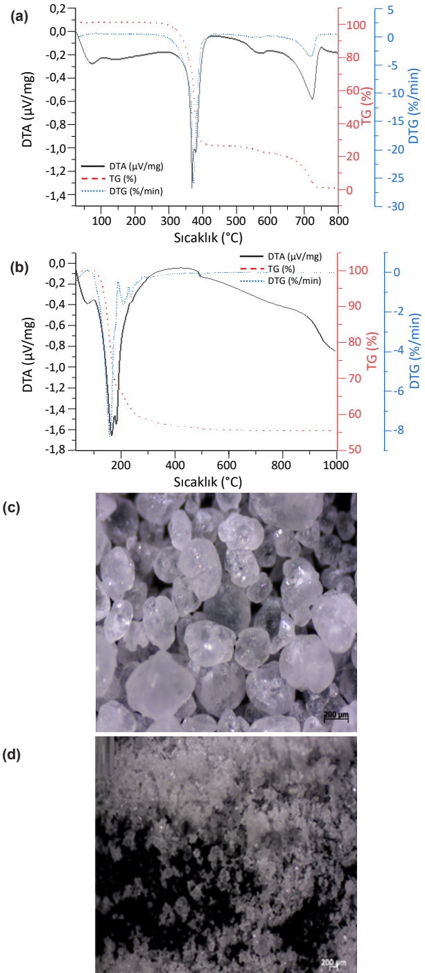
Şekil 3. a). Melamin ısı analiz grafiği, b). Borik asit ısı analiz grafiği, c) Borik asit optik mikroskop görüntüsü d) melamin optik mikroskop görüntüsü (a). Thermal analysis of the boric acid, b). Thermal analysis of the melamine, c). Optic microscope image of the boric acid d). Optic microscope image of the melamine).
