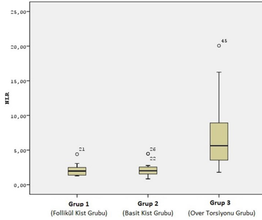
Resim 2. Grupların NLR ortalamalarına göre dağılımı ROC Curve
