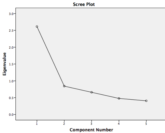
Şekil 1. Faktör yapısına ilişkin scree plot tablosu
