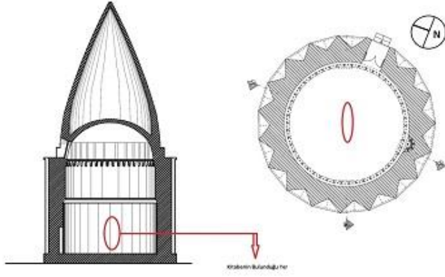
Çizim 1. Hemedan - Rezen, İmamzâde Azher Türbesi, kuzey-güney kesiti ve plan (Hemedan Kültürel Miraslar Müdürlüğü Arşivi'nden)
