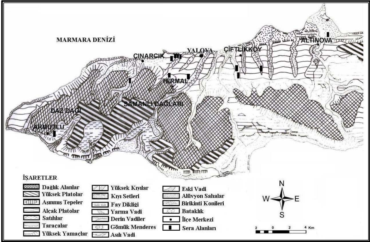
Şekil 2. Yalova İli ve çevresinin morfogrfya haritası.
