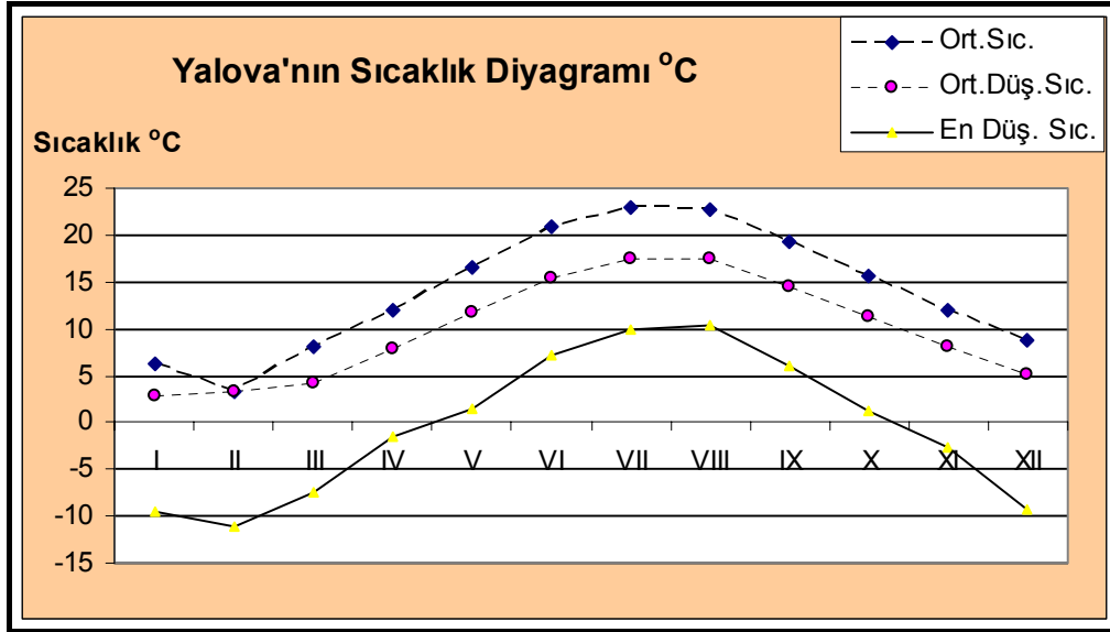
Şekil 6. Yalova'nın aylık ortalama sıcaklık diyagramı.
