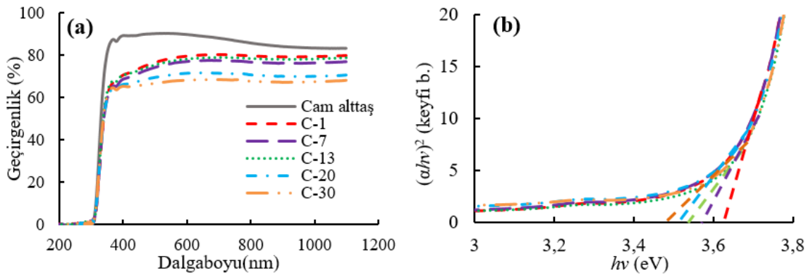
Şekil 3. Cam üzerine kaplanan Nb 2 O 5 filmlerin (a) UV-Vis geçirgenlik ve (b) (\alpha h\nu)^2 ’nin foton enerjisine göre değişimi
