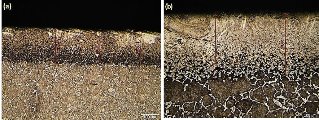
Şekil 7. 950 °C'de (a) 2,5 Saat Ve (b) 7,5 Saat Borlama Sonucu Ø11 mm Çapındaki DIN 20MnCr5 Çelik Çubukların Optik Mikroyapısı Ve Tabaka Kalınlıkları.
