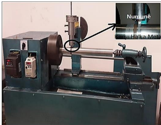
Şekil 6. Pin on ring Aşınma Test Cihazı
