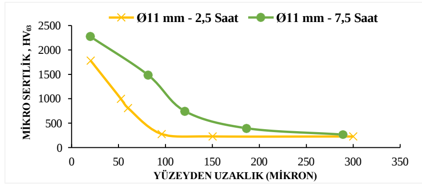
Şekil 8. Ø11 mm Çapındaki DIN 20MnCr5 Çeliğinin 950 °C Sıcaklıkta 2,5 Saat ve 7,5 Saat Kutu Borlama Sonucu Mikro Sertlik Eğrileri.
